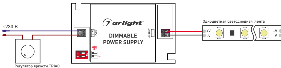
Рисунок 1. Подключение источника питания при использовании интерфейса DALI.
